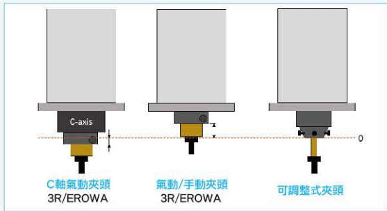
夾頭與工作台之距離
