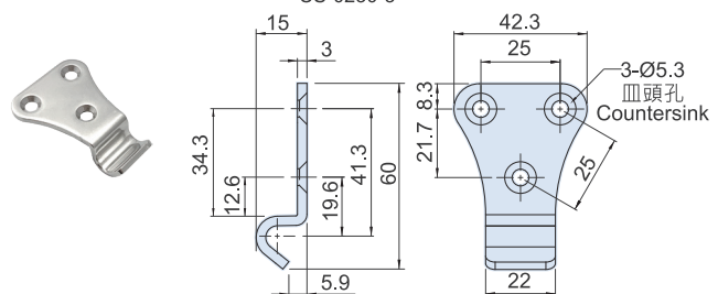
可替代鉤座 Alternative Keeper CS-0230-3
