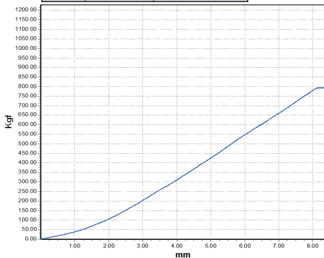
CS-5230 調整搭扣荷重測試曲線圖
