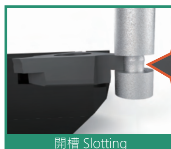
車削圓槽 Turning round groove
