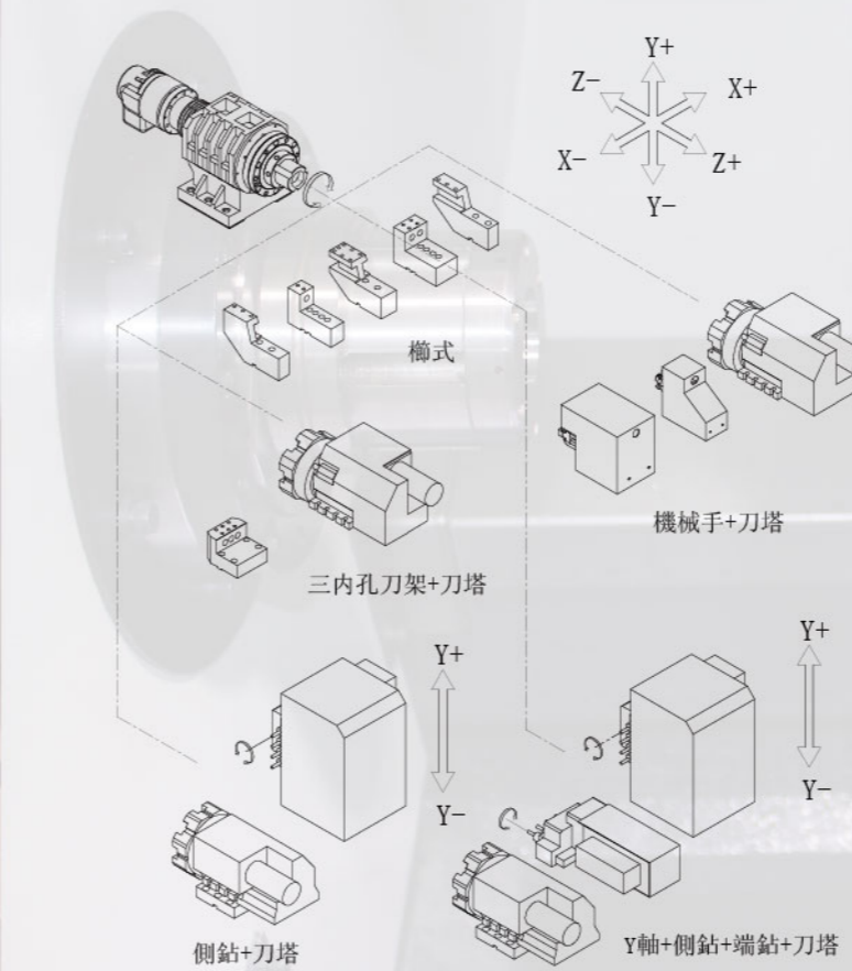
刀塔+側鑽四工位
