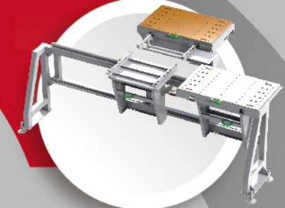
前置式工作盤交換台 Front Mounted Pallet Changer
