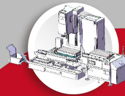
側進式自動交換工作台 Lateral Feeding (Automatic) Pallet Changer
