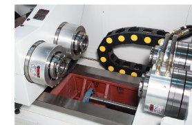
油壓夾持系統 Hydraulic clamping system
