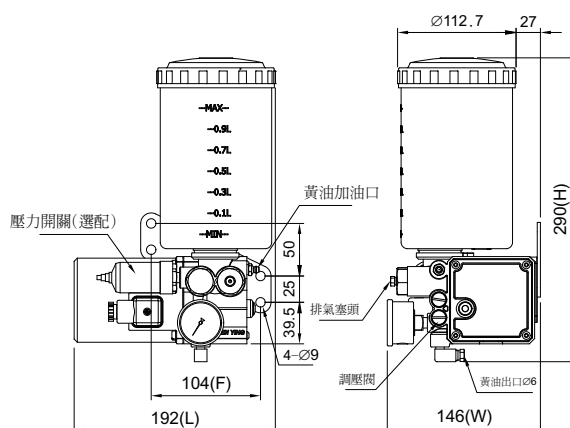
KGC-35(壓力開關為選配)外型圖
