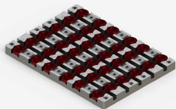
▲ 圓形油壓缸蓋加工超量產治具範例
