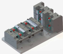
▲ 工件加工治具範例
