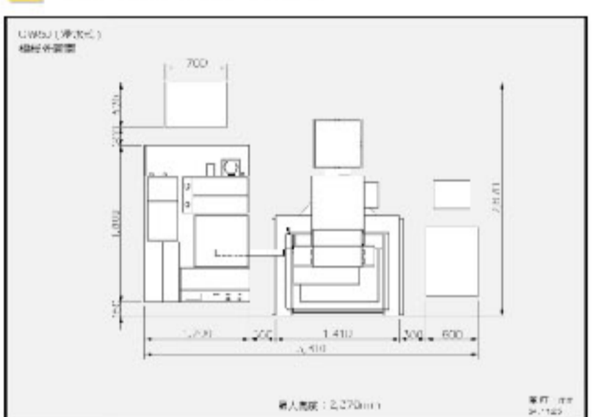
CW-50佔地面積圖
