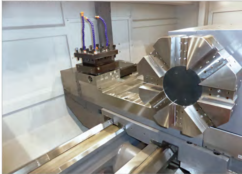
CLT-100SPV(動力刀塔)
