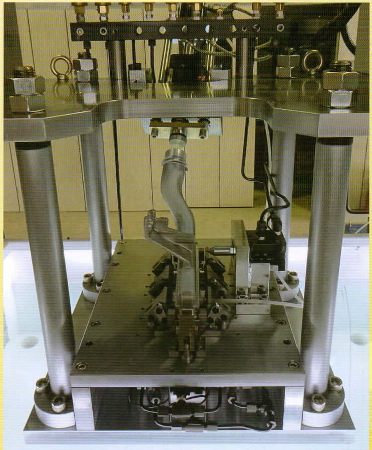
測漏機用治具
