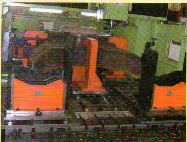
手動治具 Manual Fixtures
