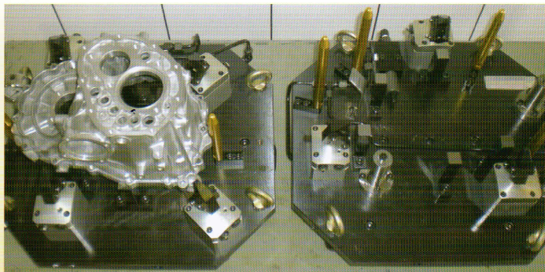
交換台用油壓治具 Hydraulic Fixtures
