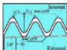
BSPT 55° 英制錐管螺紋 55°
