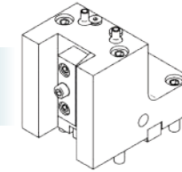
外徑刀座 C Turning tool holder
