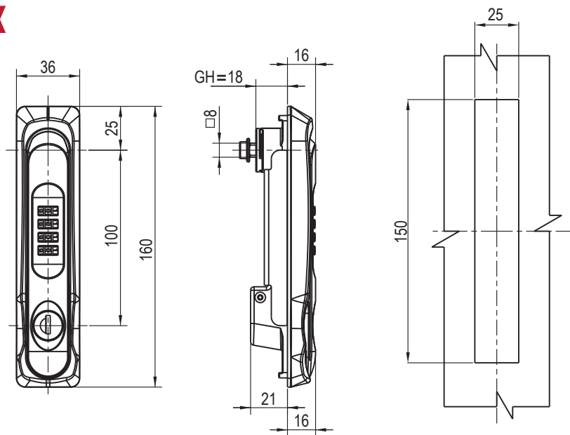
開孔尺寸 Panel Cutout
