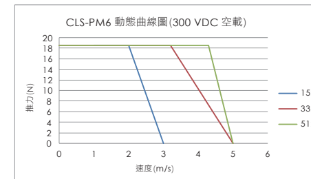
本圖是以5m/s為最大速度限制，若需更高速度或特殊需求，請聯絡cpc
