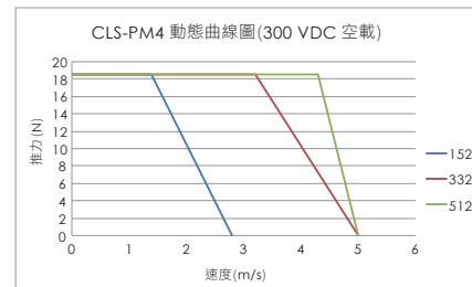
本圖是以5m/s為最大速度限制，若需更高速度或特殊需求，請聯絡cpc
